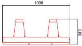
A型 面図
